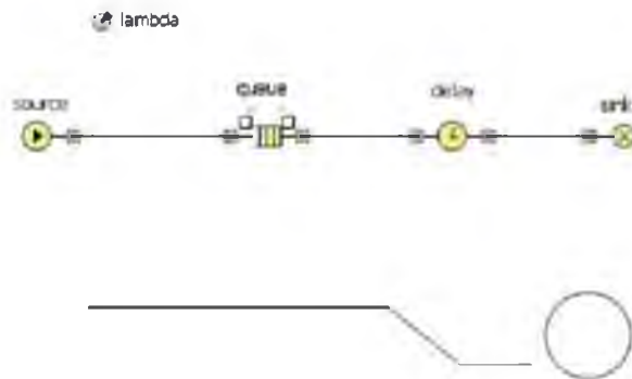
Рис.3.15. Анимация очереди
