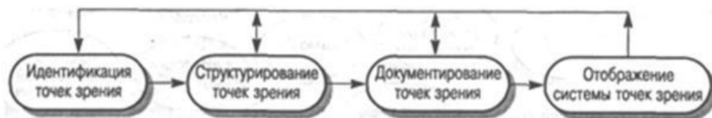
Рис. 3. Метод VORD
