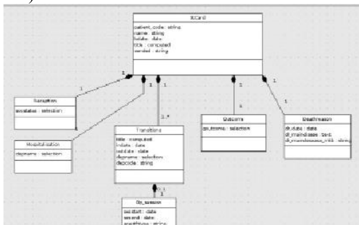
Рис. 1. Диаграмма классов
